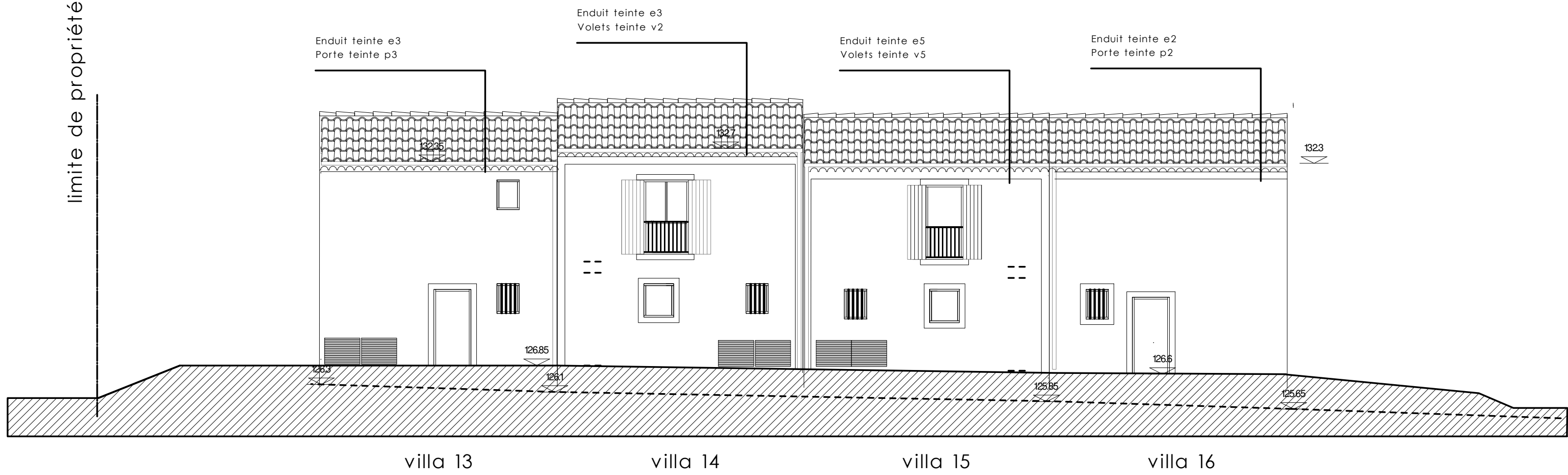
FACADES NORD
