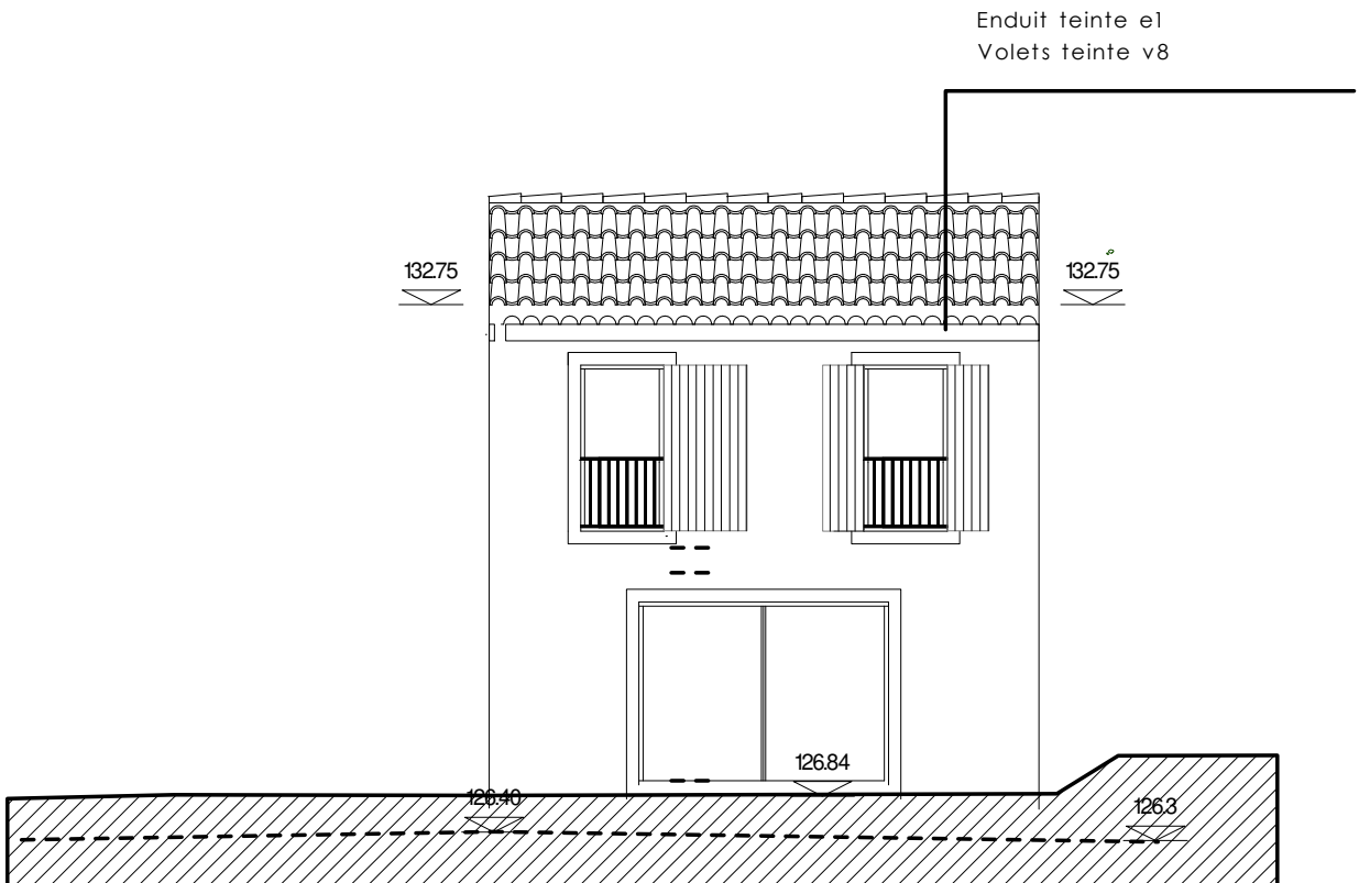
FACADES NORD VILLA 12
