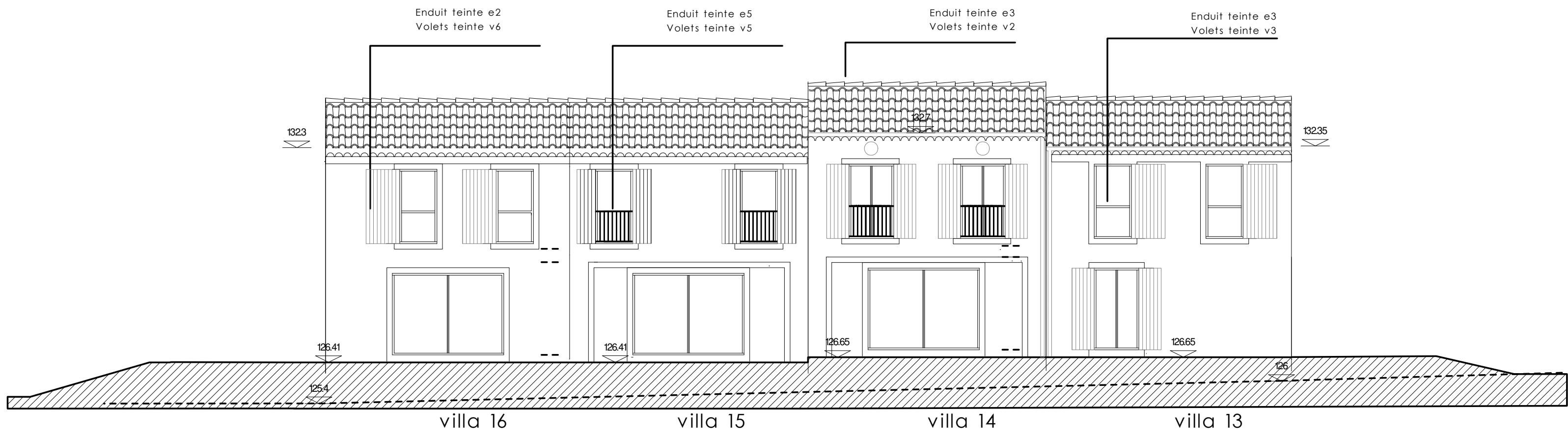
FACADES SUD
