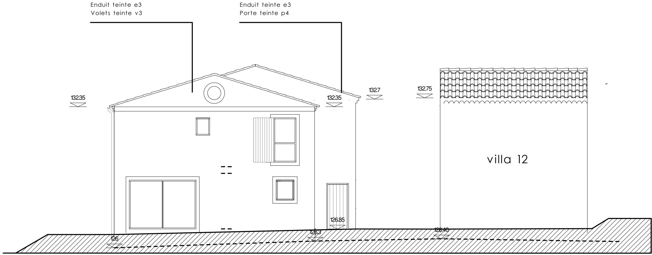
FACADE EST VILLA 13
