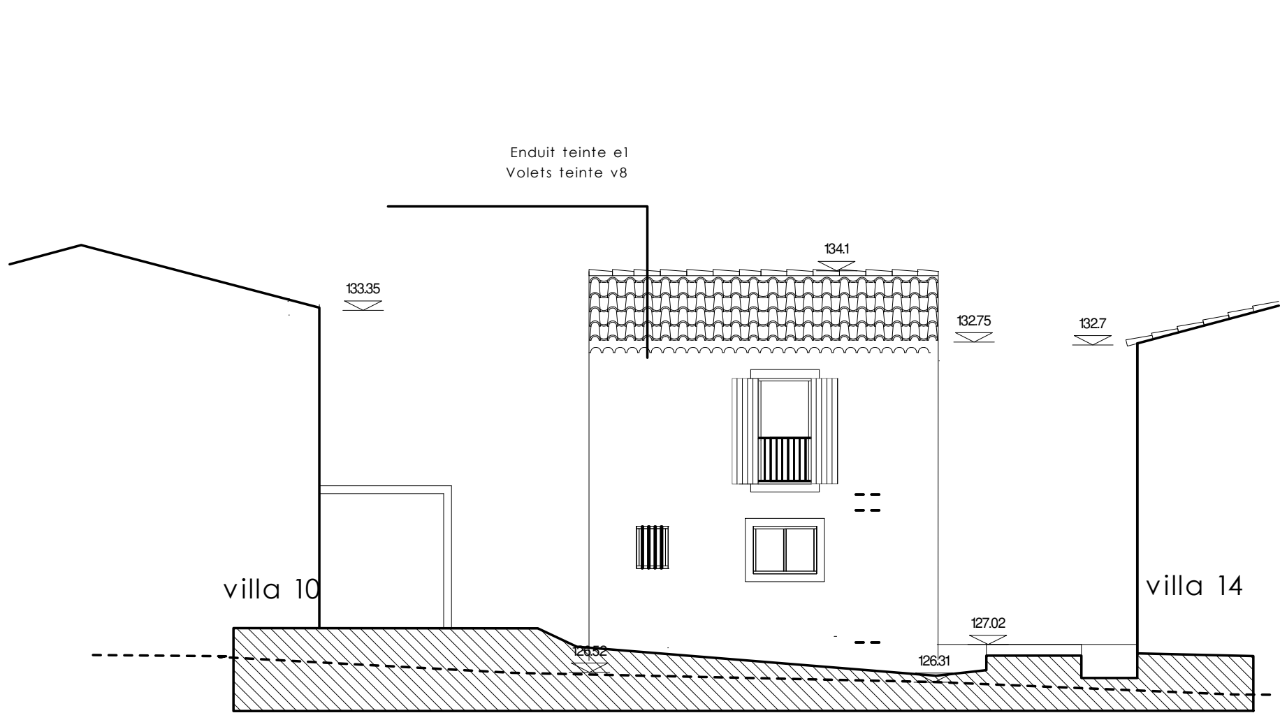
FACADE OUEST VILLA 12
